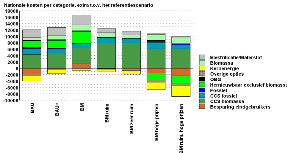
Figuur 2: Nationale kosten naar optieccategorie, BAU, BAU+, Blue map en varianten
