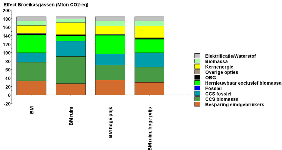
Figuur 8: Reducties per categorie voor verschillende energieprijzaanname
