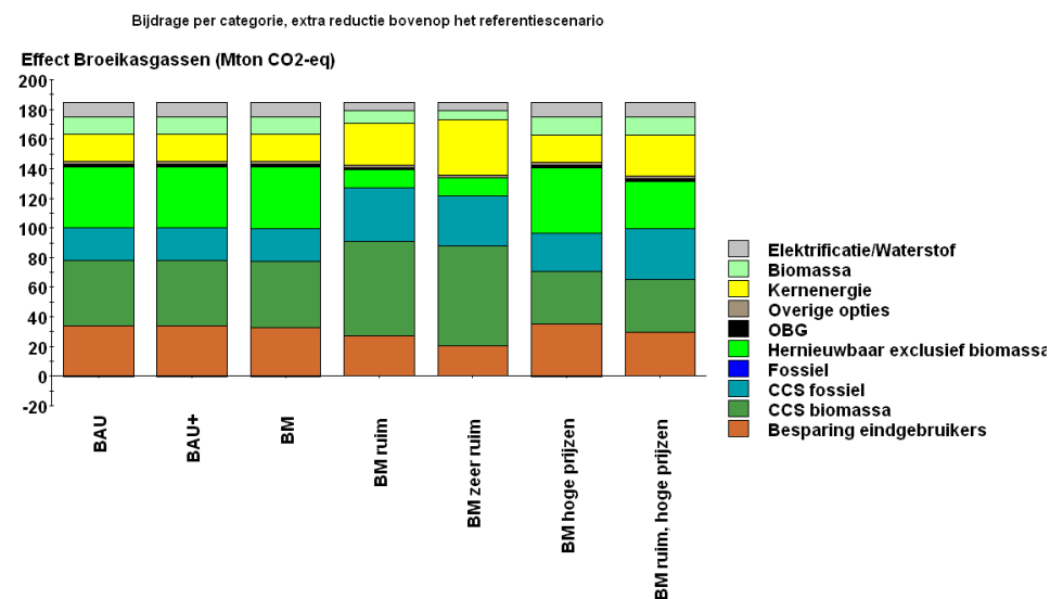
Figuur 3: Emissiereductie naar optieccategorie, BAU, BAU+, Blue map en varianten
