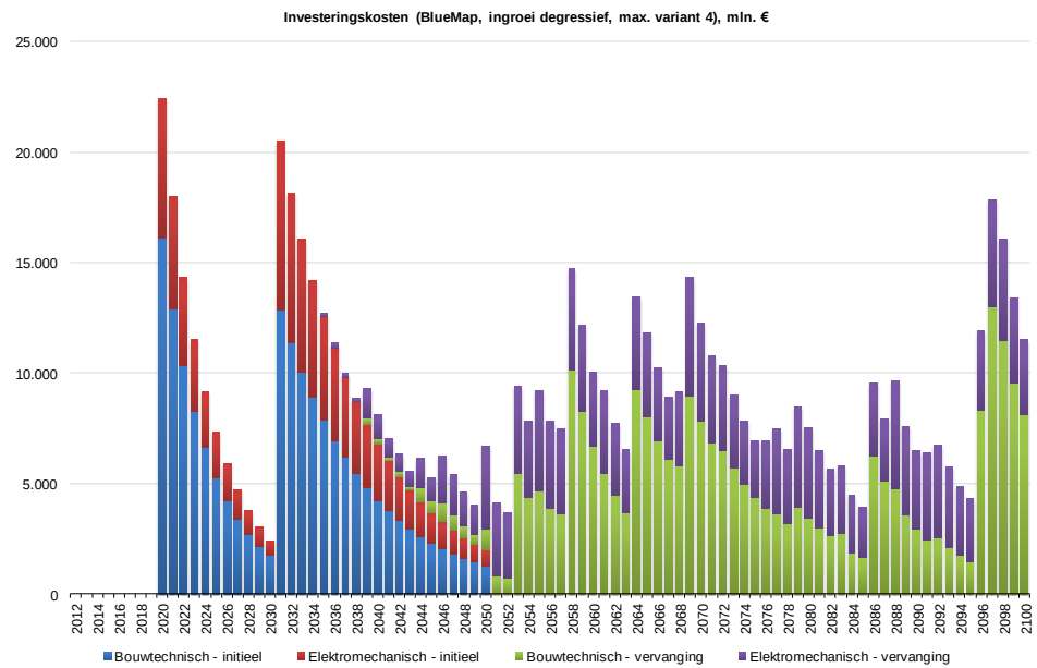
Figuur 24: Een versneld investeringstempo (degressieve curve)
