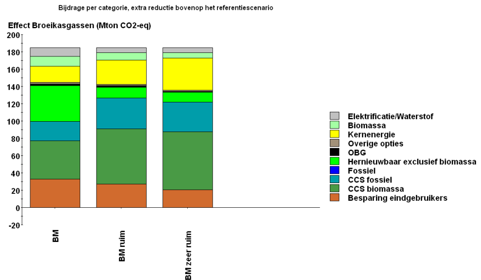
Figuur 7: Reducties per categorie voor verschillende potentieelaannames
